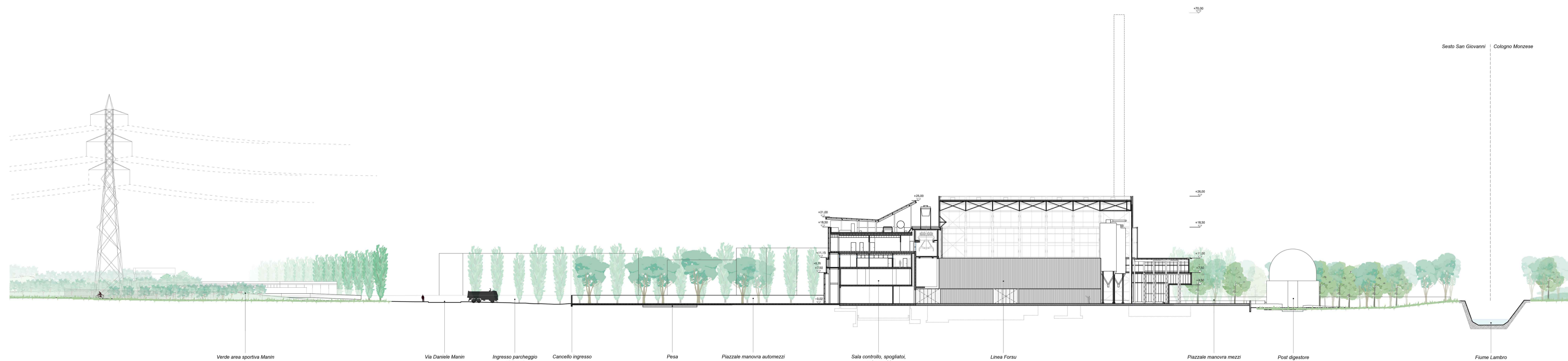
PROGETTO - SEZIONI GENERALI 3 - 3
